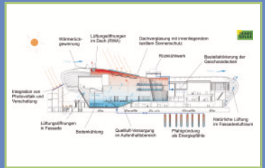
Schematische Darstellung des Energiekonzeptes im Klimahaus® Bremerhaven 8° Ost:
