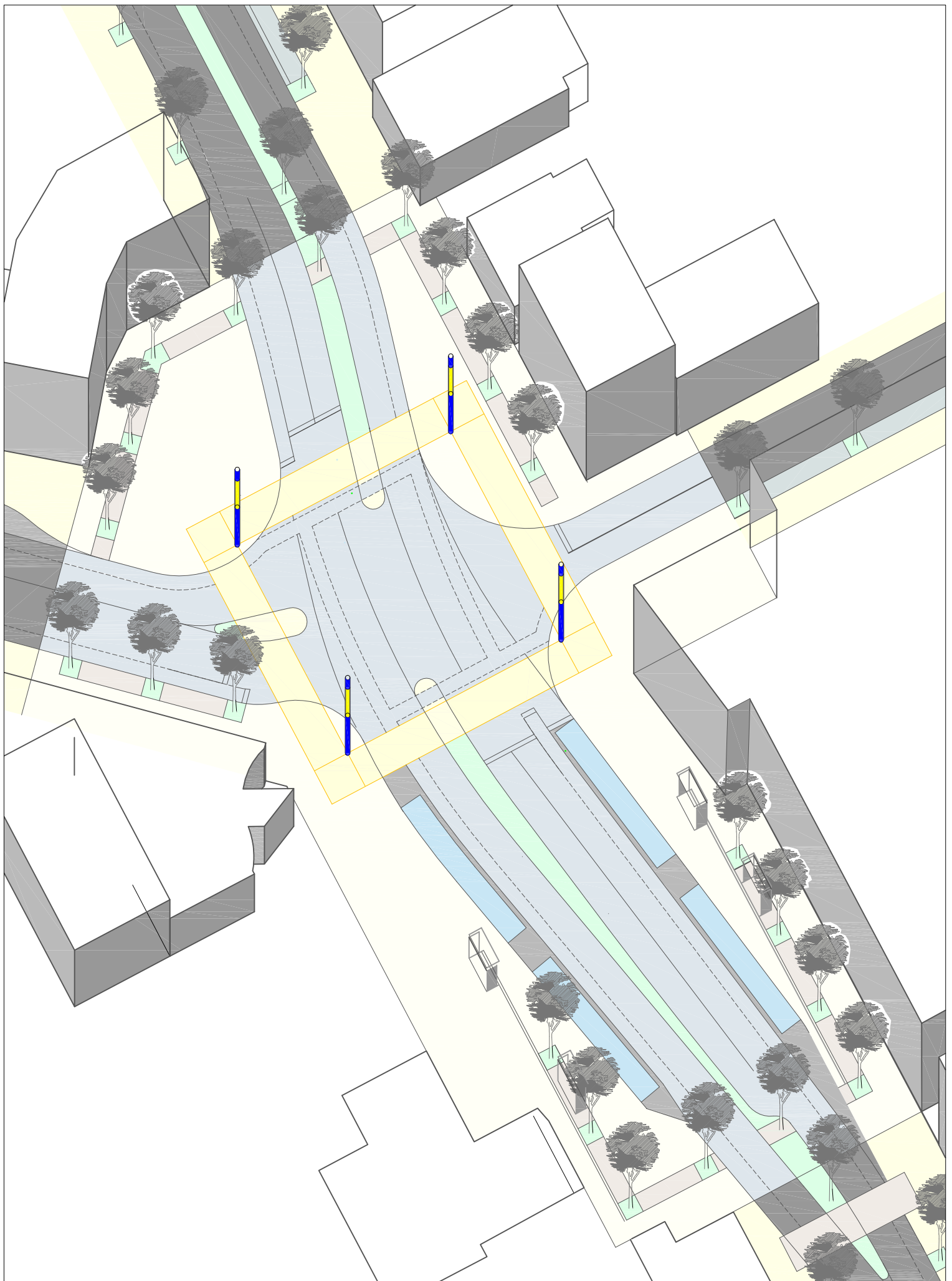
Umgestaltung Weserstraße/Lindenallee Ortsteil Wulsdorf, Stadt Bremerhaven Isometrie - ABSCHNITT MITTE - VORZUGSVARIANTE V 1 Maßstab: 1: 500 @ DIN A4 / Stand 12.09.2018
